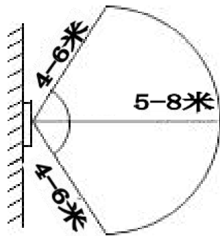
(墙壁安装图示)
