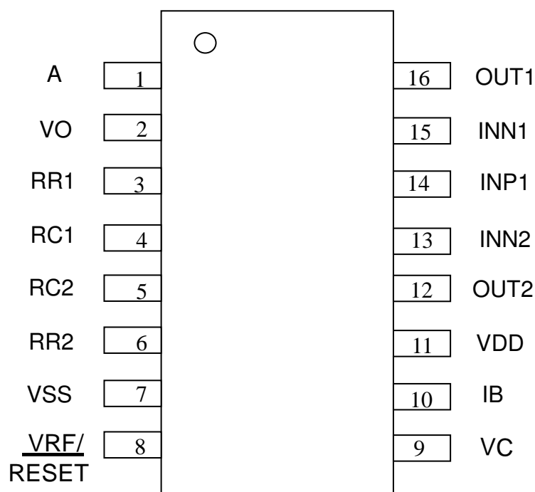
图 1 : SP013兼容 (BISS0001)外引线连接图
